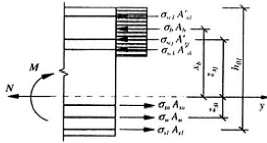
Hình 25 - Sơ đồ nội lực và biểu đồ ứng suất trong tiết diện thẳng góc với trục dọc cấu kiện có đặt nhiều lớp cốt thép khi tính toán theo biến dạng
