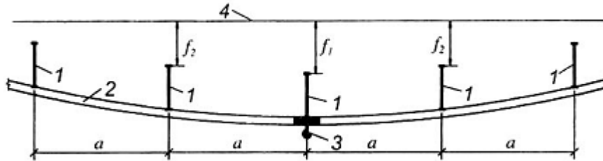
Hình C1 - Sơ đồ xác định các giá trị l ( l_1, l_2, l_3 ), khi có tường ngăn giữa các tầng chịu lực
